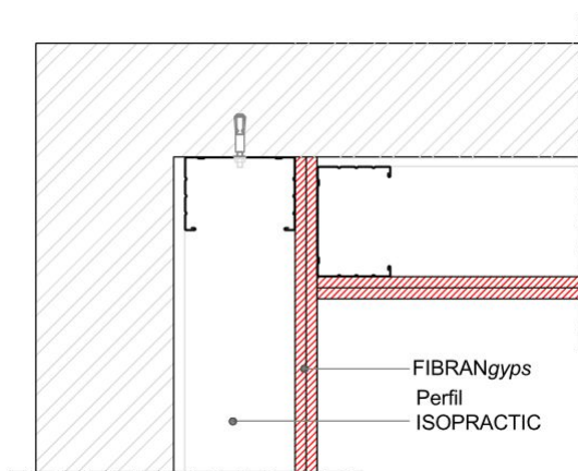
Det. 3 CONEXIÓN A "L"
