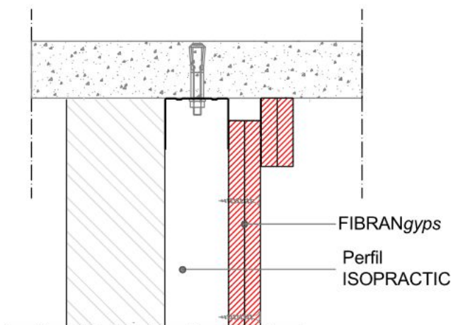
Det. 4 JUNTA PARA DILATACIÓN VERTICAL
