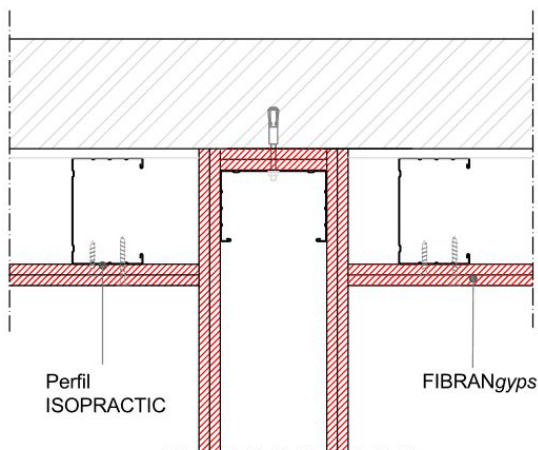
Det. 1 CONEXIÓN A LA PARED
