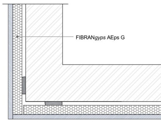
Det. 3 CONEXIÓN A "L" EXTERIOR
