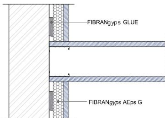
Det. 1 CONEXIÓN A LA PARED
